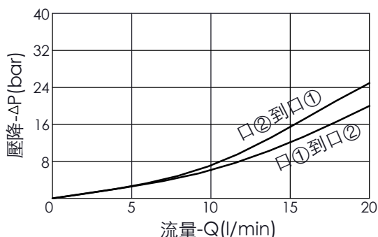
性能曲線
